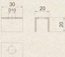
7. Assembly piece. Pieza de unión. Pièce de raccordement.
