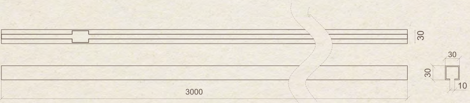
4. Ceiling profile. (Curved version also available) Perfil techo. (Versión curvada también disponible). Profil de plafond. (Version courbée également disponible)
