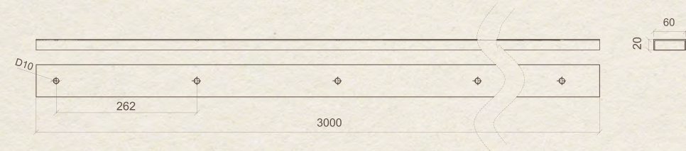
3. Floor profile. (Curved version also available) Perfil de apoyo. (Versión curvada también disponible). Profil du sol. (Version courbée également disponible)
